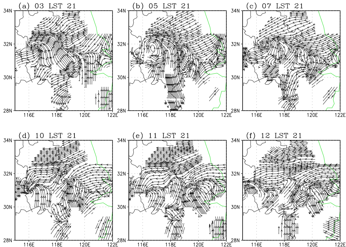
Fig. 7. Surface streamlines on 21 June 2002, (a) 0300 LST, (b) 0500 LST, (c) 0700 LST, (d) 1000 LST, (e) 1100 LST, (f) 1200 LST.
