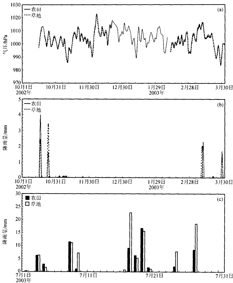
图2 日降雨量及日平均气压的逐日变化 (a) 日平均气压; (b) 2002年10月1日~2003年3月30日降雨量; (c) 2003年7月1日~31日降雨量
